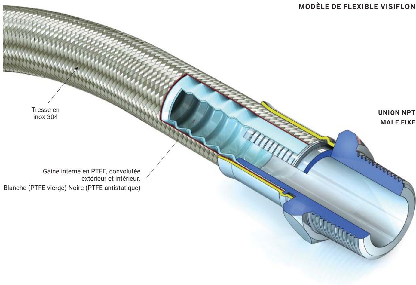
MODÈLE DE FLEXIBLE VISIFLON
